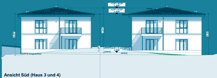
Ansicht Süd (Haus 3 und 4)
