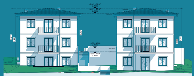
Ansicht Nord (Haus 1 und 2)
