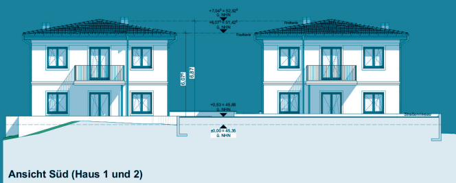
Ansicht Süd (Haus 1 und 2)
